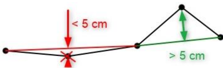
Rys. 2. Zasada redukcji załamań (werteksów) poziomic.
