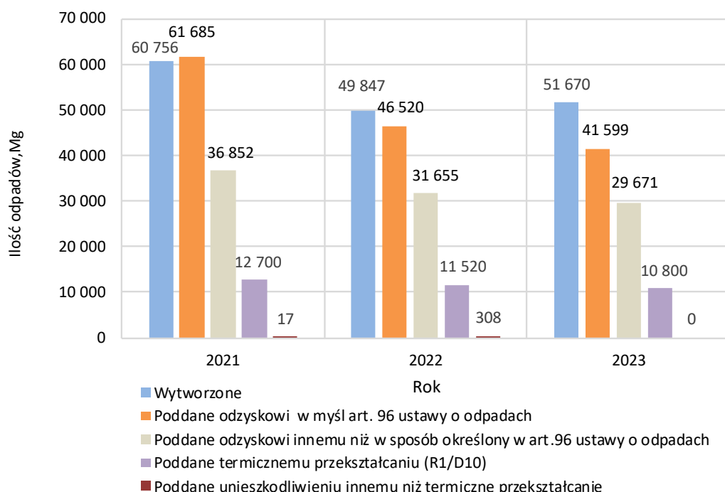
Rysunek 22. Masa komunalnych osadów ściekowych wytworzonych, poddanych procesom odzysku oraz unieszkodliwiania na terenie województwa opolskiego w latach 2021–2023 75
