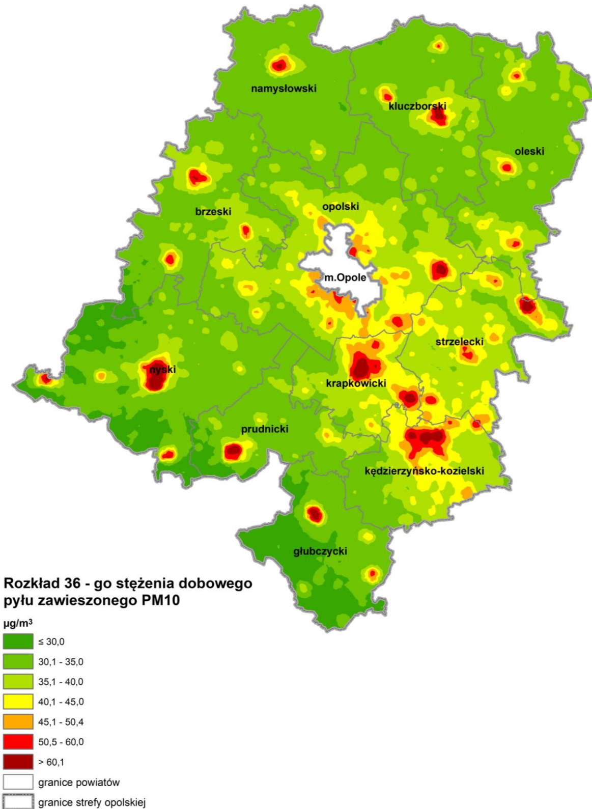
Rysunek 11. Rozkład stężeń 24-godzinnych pyłu zawieszonego PM10 w strefie opolskiej wyrażone jako maksymalne 36-te stężenie dobowe w roku bazowym 2016 (źródło: opracowanie własne na podstawie wyników modelowania modelem CALPUFF dla 2016 r.).
