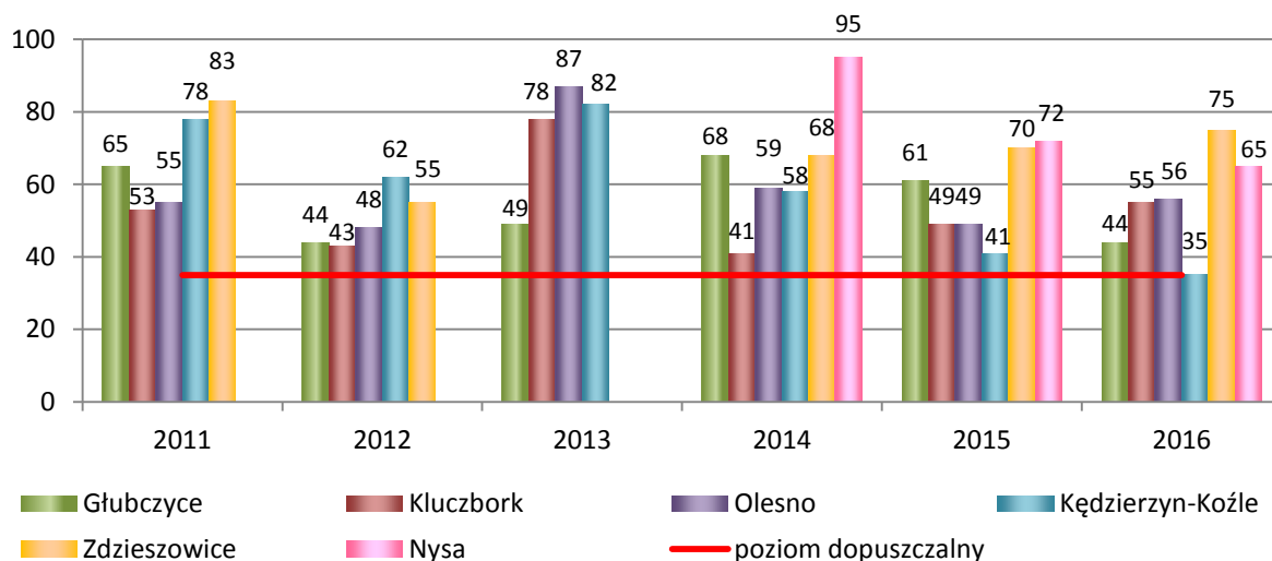
Rysunek 22. Ilość dni z przekroczeniem dopuszczalnego poziomu 24-godzinnego pyłu zawieszonego PM10 w strefie opolskiej w latach 2011-2016 (źródło: opracowanie własne na podstawie danych WIOŚ).
