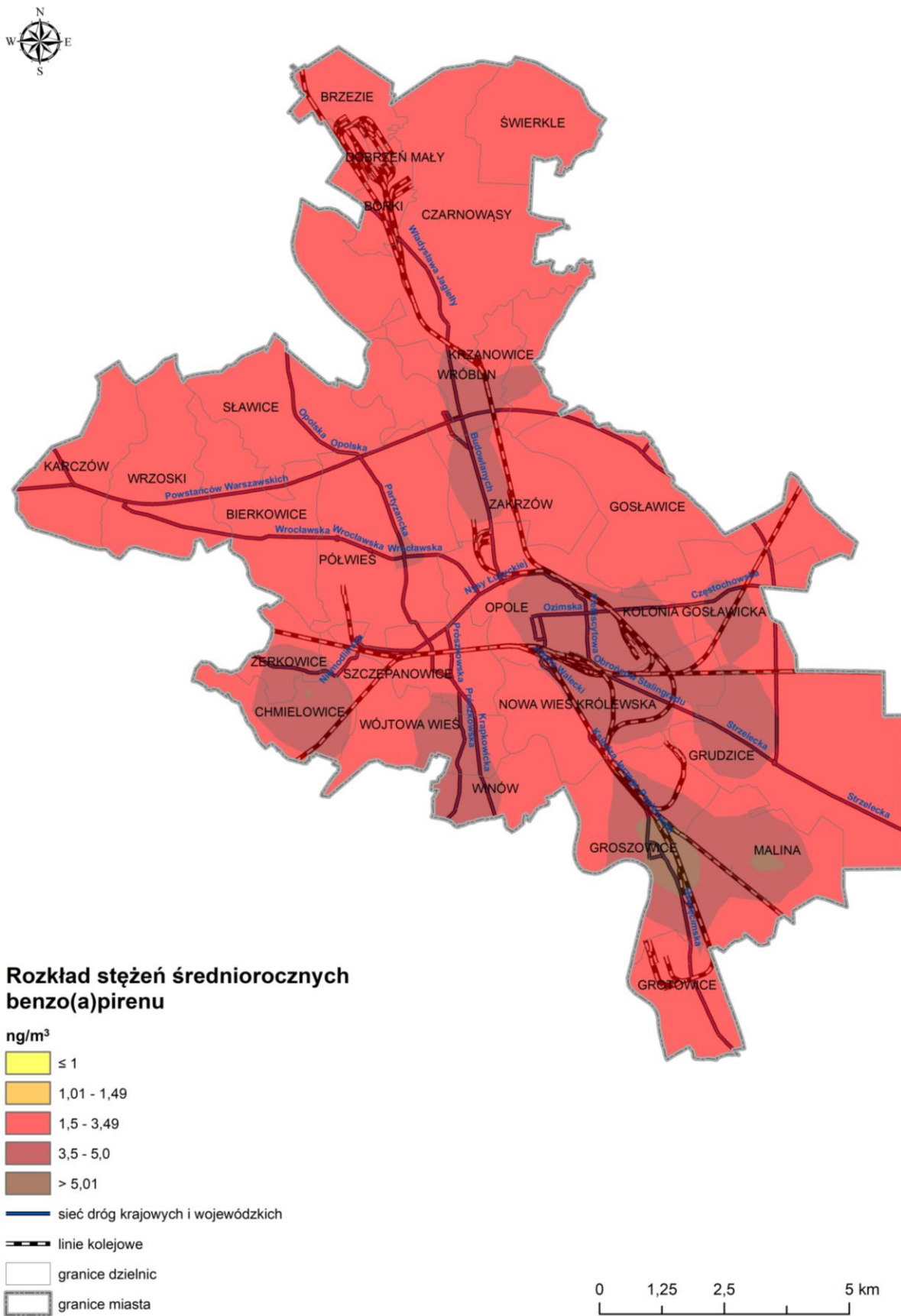
Rysunek 9. Rozkład stężeń średniorocznych benzo(a)pirenu w strefie miasto Opole w roku bazowym 2016 (źródło: opracowanie własne na podstawie wyników modelowania modelem CALPUFF dla 2016 r.).
