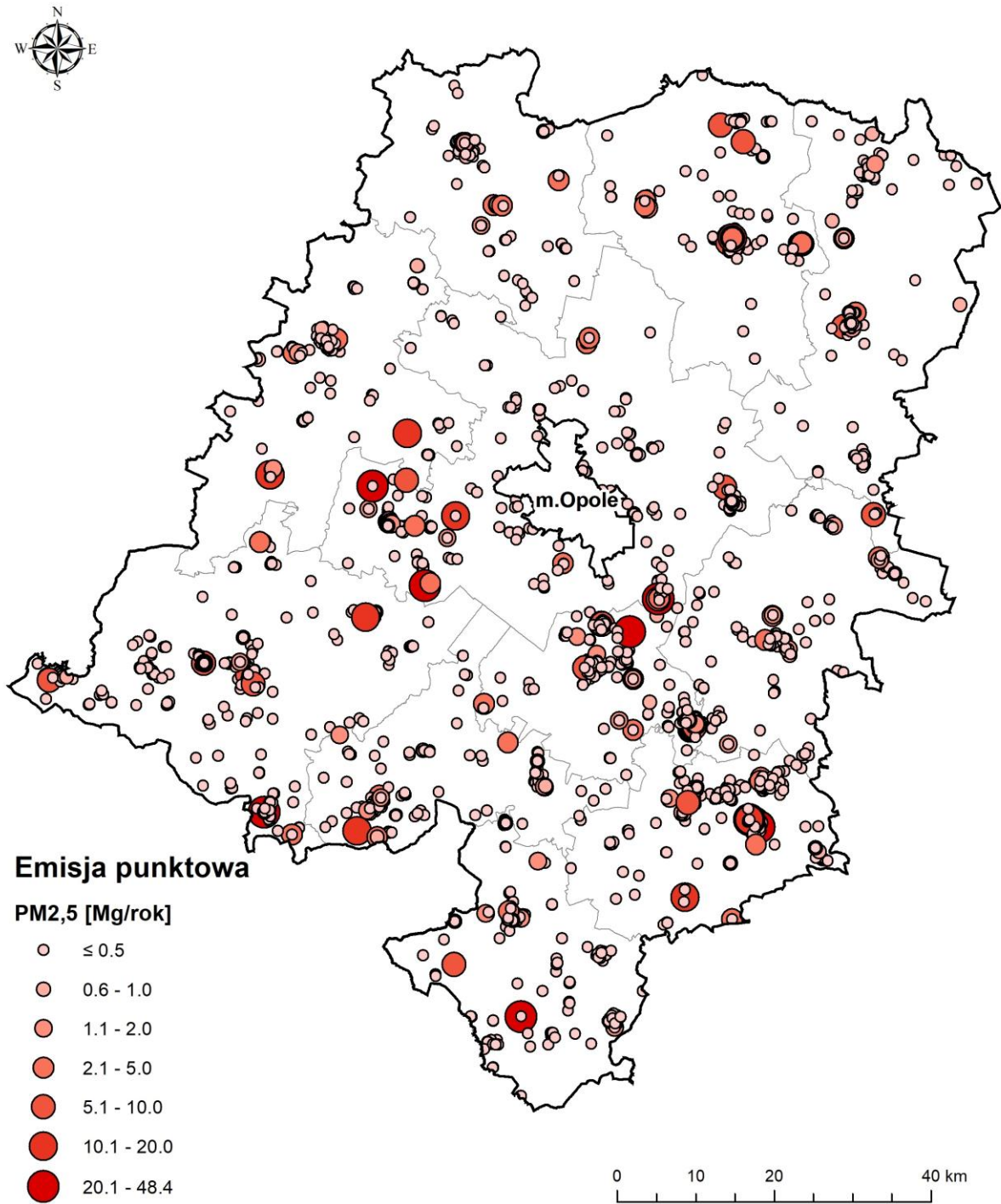
Rysunek 54. Rozkład emisji punktowej pyłu zawieszonego PM2,5 w roku 2016 na terenie strefy opolskiej (źródło: opracowanie własne).
