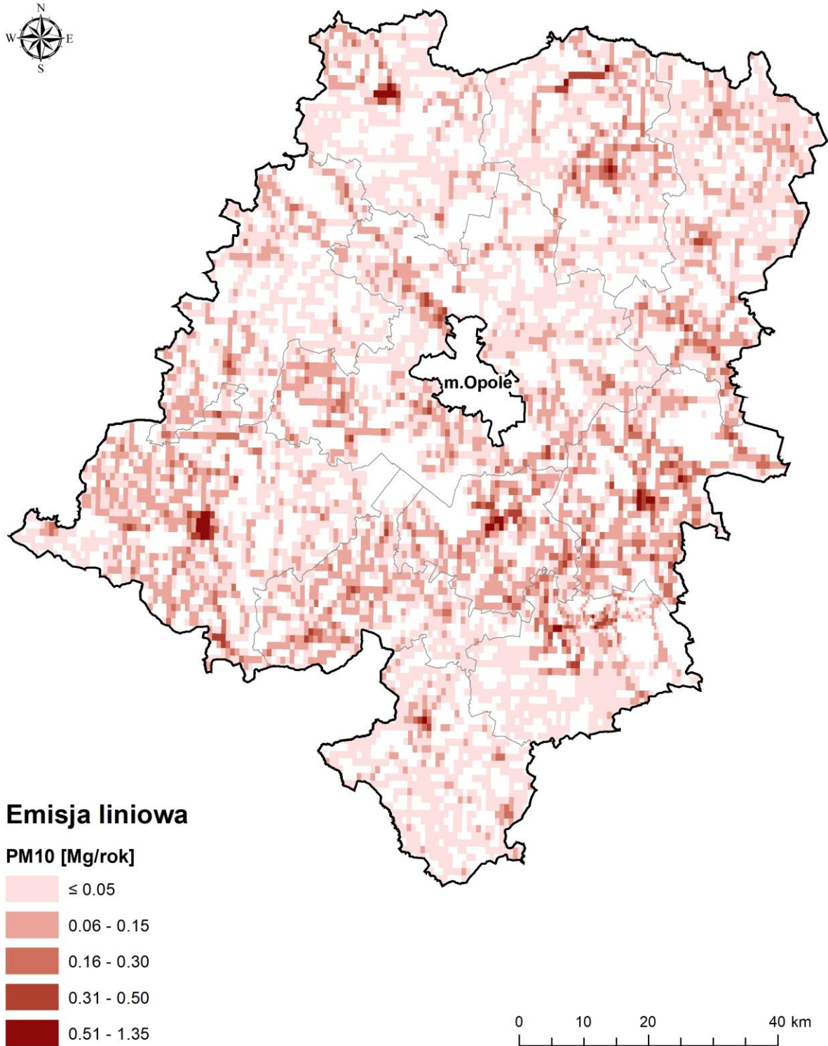
Rysunek 73. Rozkład emisji liniowej pyłu zawieszzonego PM10 z dróg powiatowych i gminnych w roku 2016 na terenie strefy opolskiej (źródło: opracowanie własne).
