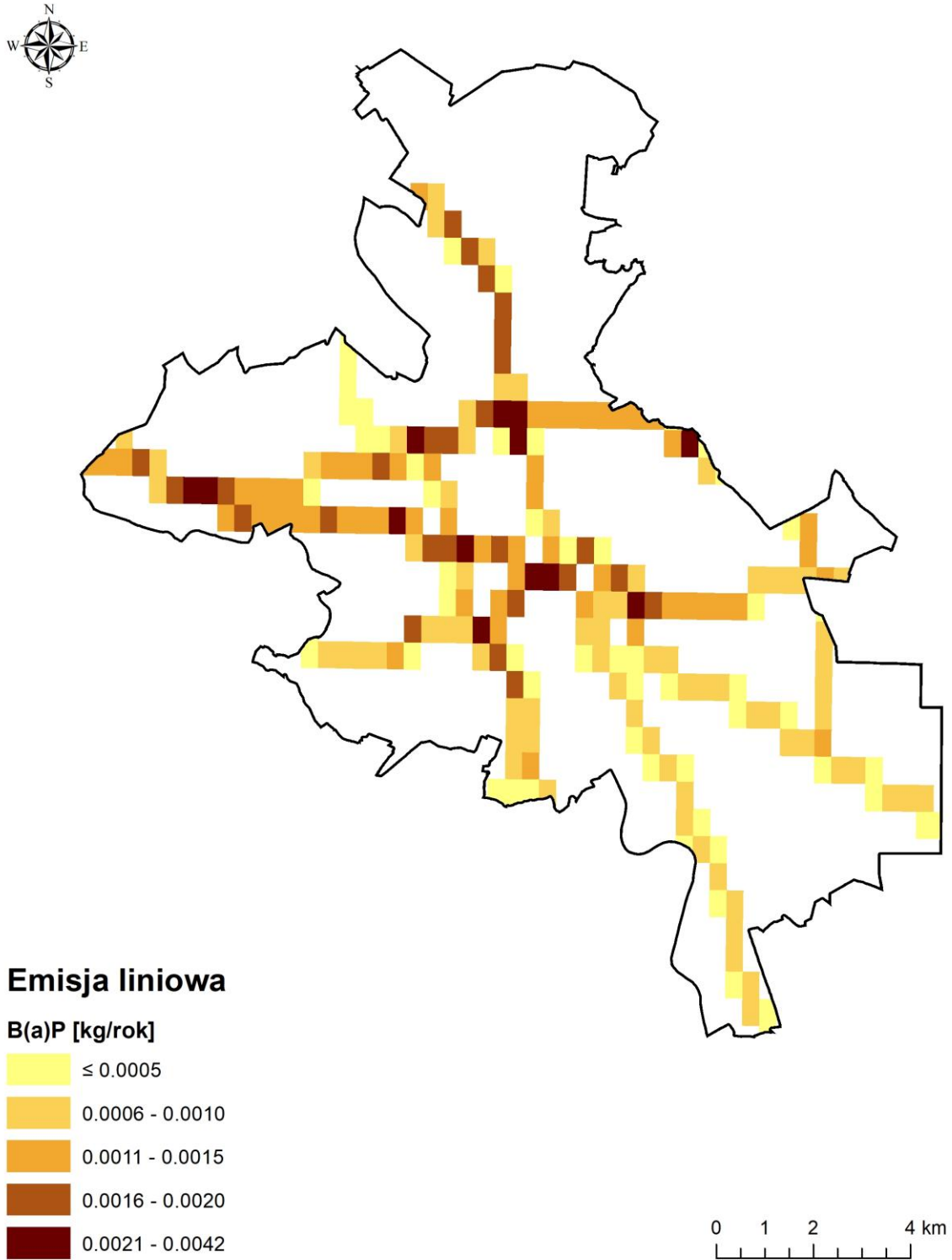
Rysunek 66. Rozkład emisji liniowej benzo(a)pirenu z dróg krajowych i wojewódzkich w roku 2016 na terenie strefy miasto Opole (źródło: opracowanie własne).
