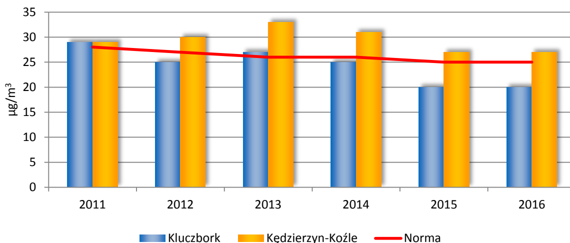
Rysunek 24. Wyniki pomiarów średniorocznych pyłu zawieszonego PM2,5 w latach 2011-2016 na terenie strefy opolskiej (źródło: opracowanie własne na podstawie danych WIOŚ).
