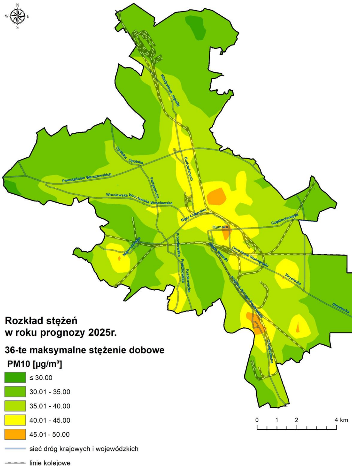
Rysunek 37. Rozkład stężeń 24-godzinnych wyznaczonych jako 36-te maksymalne stężenie pyłu zawieszonego PM10 w strefie miasto Opole w roku prognozy 2025 (źródło: opracowanie własne na podstawie wyników modelowania modelem CALPUFF dla 2016 r.).
