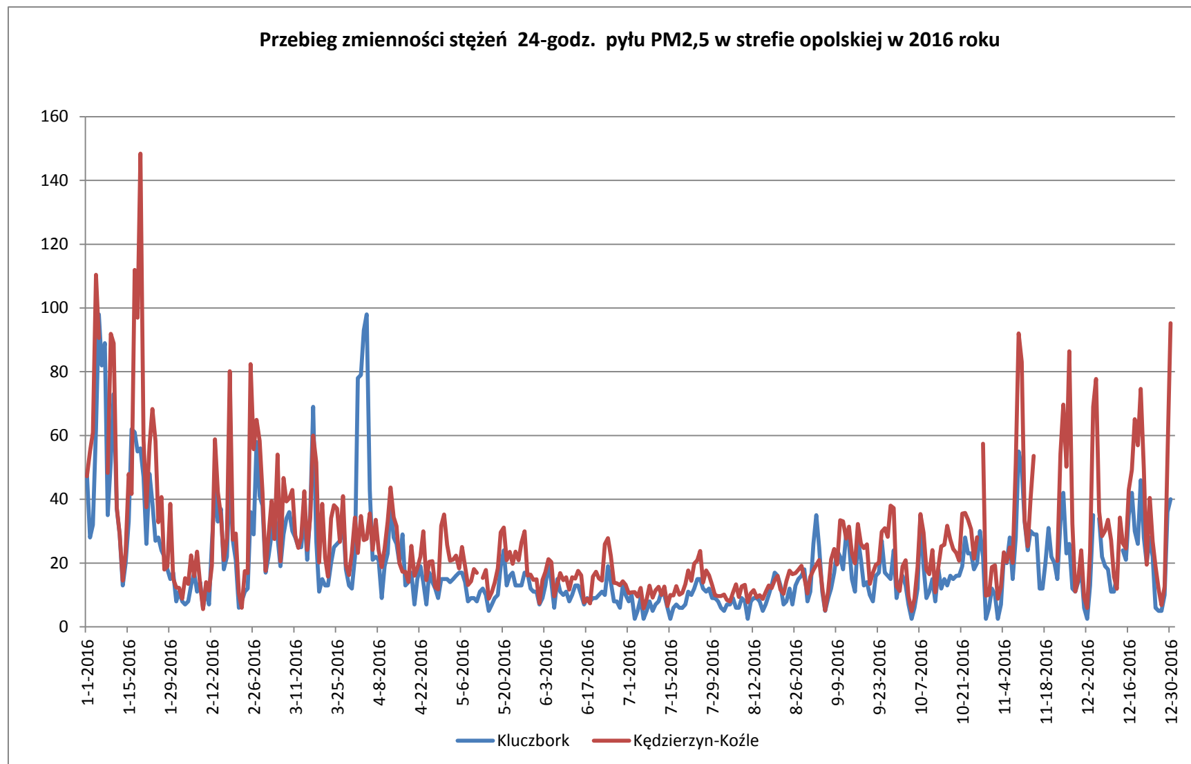
Rysunek 25. Rozkład stężeń pyłu zawieszonego PM 2,5 w roku 2016 na stacjach pomiarowych w strefie opolskiej (źródło: opracowanie własne na podstawie danych WIOŚ).
