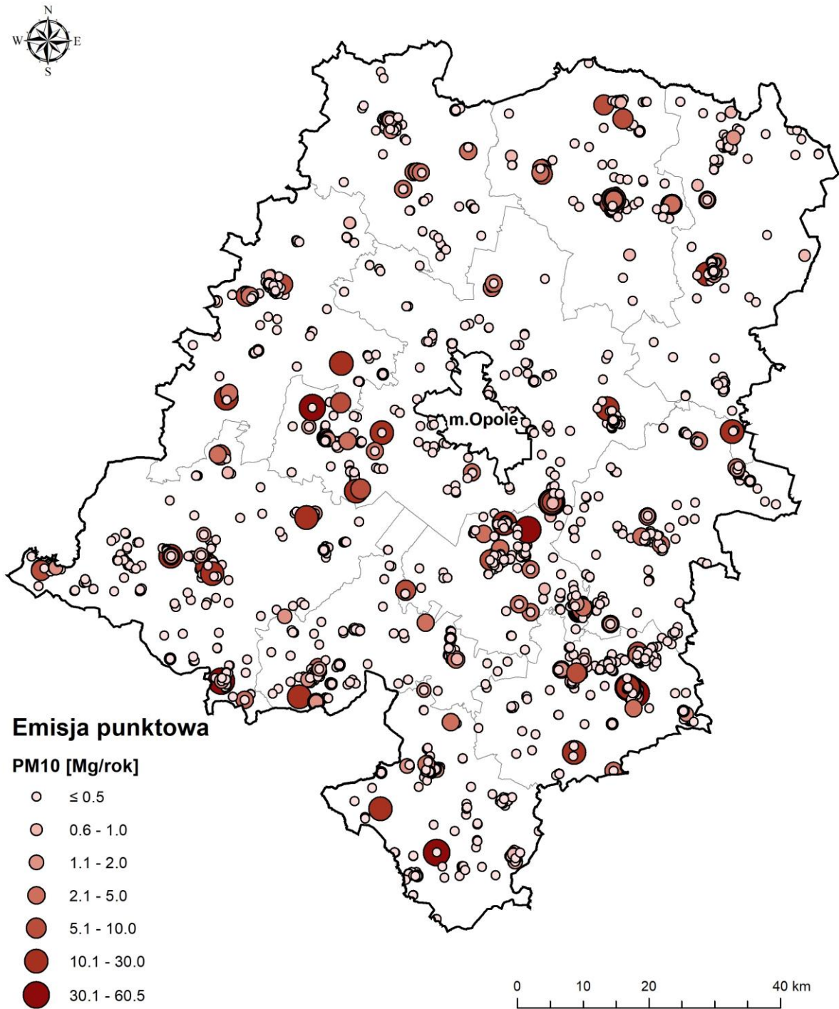
Rysunek 53. Rozkład emisji punktowej pyłu zawieszono PM10 w roku 2016 na terenie strefy opolskiej (źródło: opracowanie własne).
