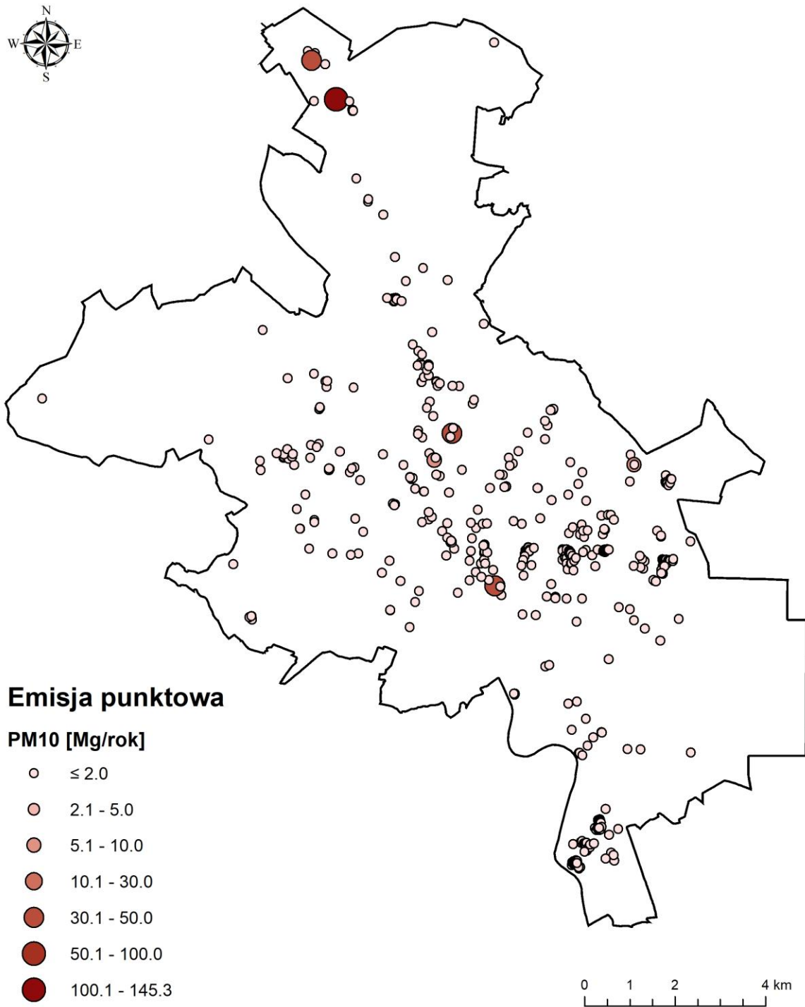
Rysunek 51. Rozkład emisji punktowej pyłu zawieszonoego PM10 w roku 2016 na terenie strefy miasto Opole (źródło: opracowanie własne).
