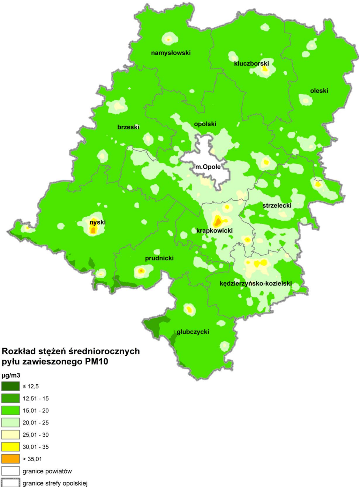
Rysunek 10. Rozkład stężeń średniorocznych pyłu zawieszonego PM10 w strefie opolskiej w roku bazowym 2016 (źródło: opracowanie własne na podstawie wyników modelowania modelem CALPUFF dla 2016 r.).
