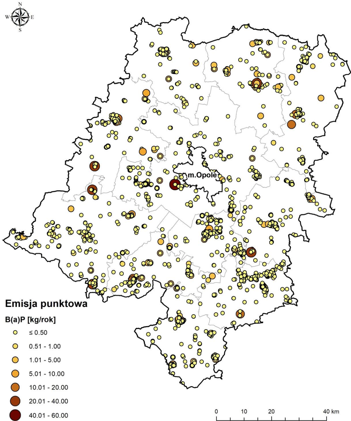
Rysunek 55. Rozkład emisji punktowej benzo(a)pirenu w roku 2016 na terenie strefy opolskiej (źródło: opracowanie własne).
