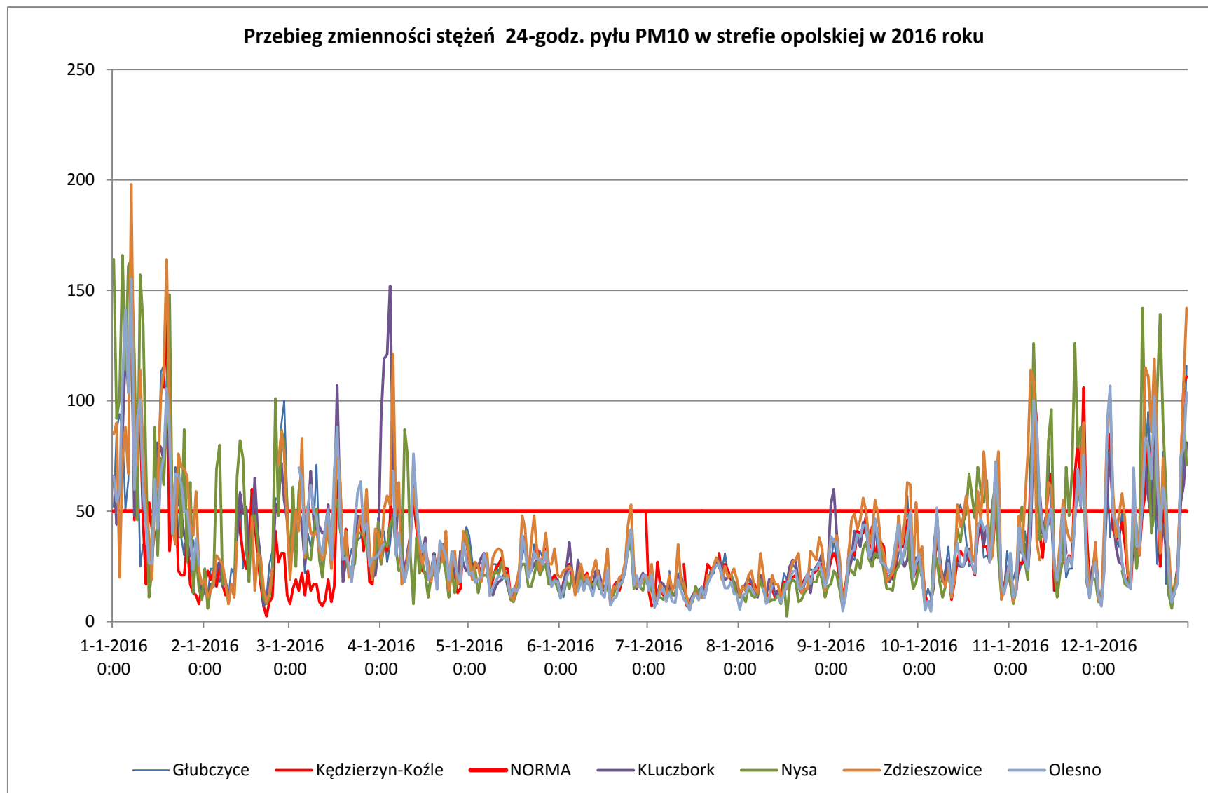
Rysunek 23. Rozkład stężeń pyłu zawieszzonego PM10 w roku 2016 na stacjach pomiarowych w strefie opolskiej (źródło: opracowanie własne na podstawie danych WIOŚ).
