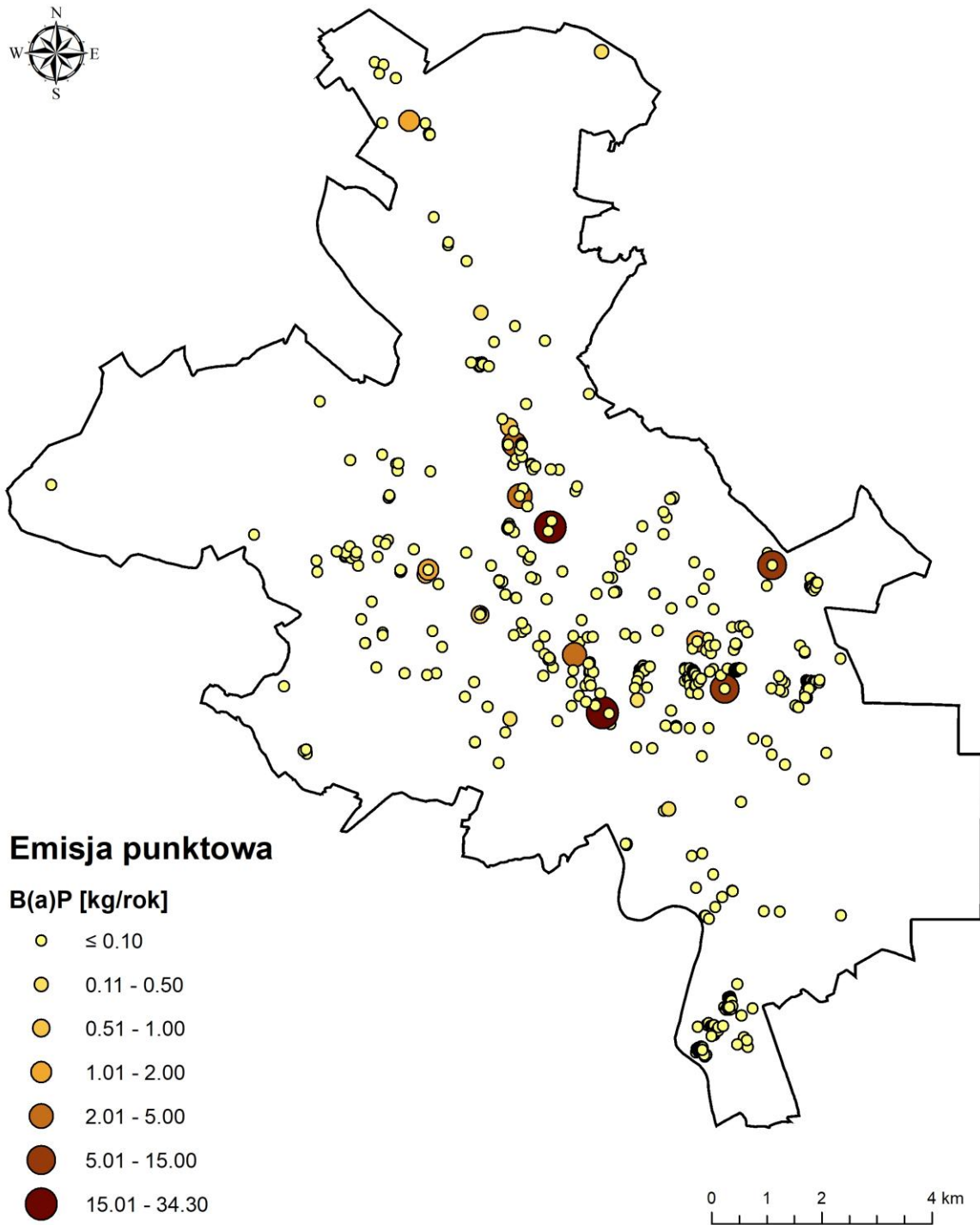
Rysunek 52. Rozkład emisji punktowej benzo(a)pirenu w roku 2016 na terenie strefy miasto Opole (źródło: opracowanie własne).
